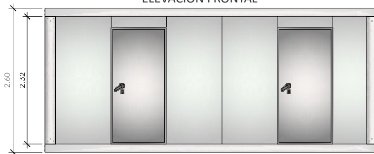
ELEVACIÓN FRONTAL
