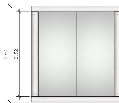
ELEVACIÓN LATERAL (derecha e izquierda)
