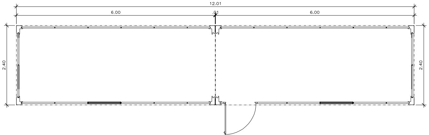
PLANTA DE DISTRIBUCIÓN
